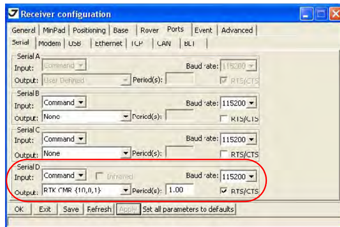
Рисунок 3-10. Закладка Ports
