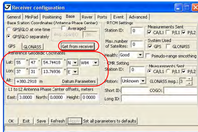
Рисунок 3-9. Закладка Base
