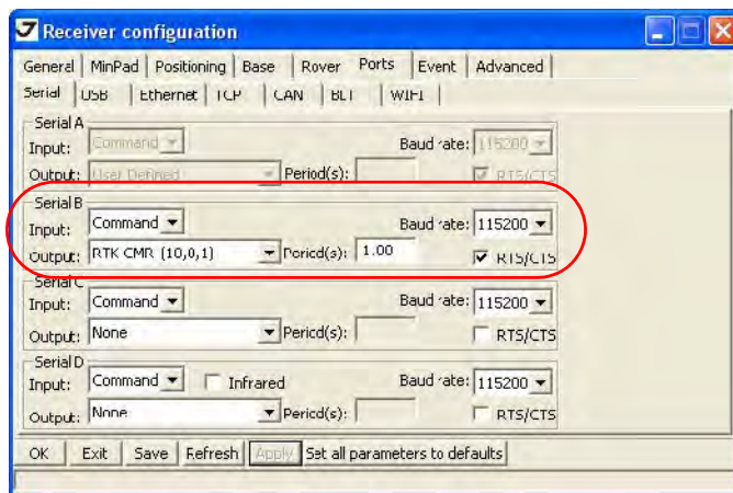
Рисунок 3-6. Закладка Ports
