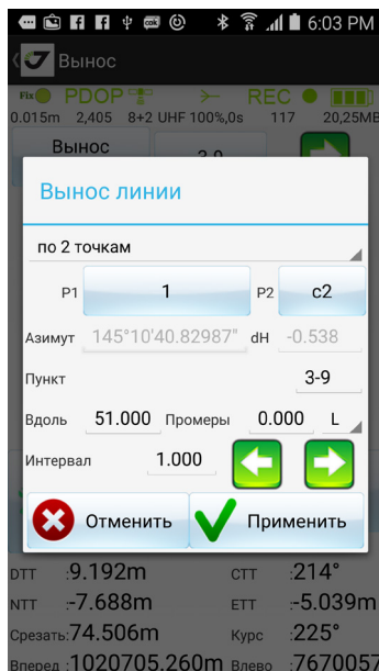
Рисунок 47. Задание точки относительно линии
