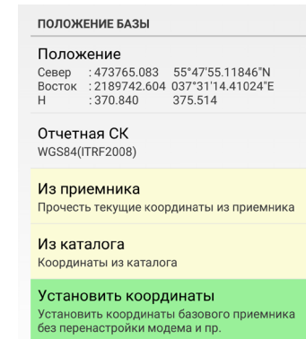
Рисунок 36. Положение базы
