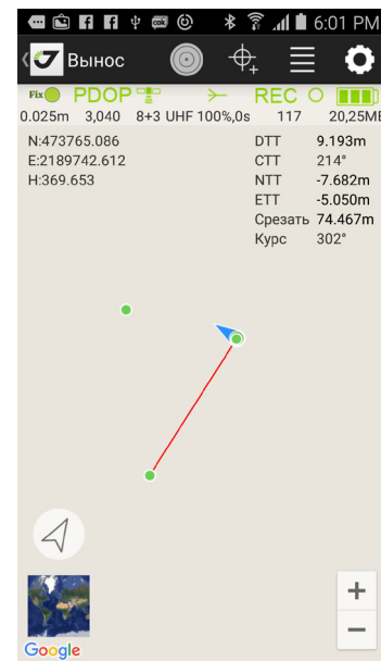
Рисунок 46. Экран выноса в натуру
