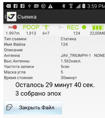
Пост-процессорная съемка
