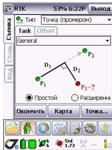
Рисунок 4-3. Съёмка точки (промером)
