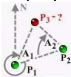
Рисунок 6-11. Угол-Угол
