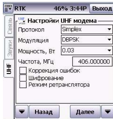
Рисунок 8-10. UHF modem settings
